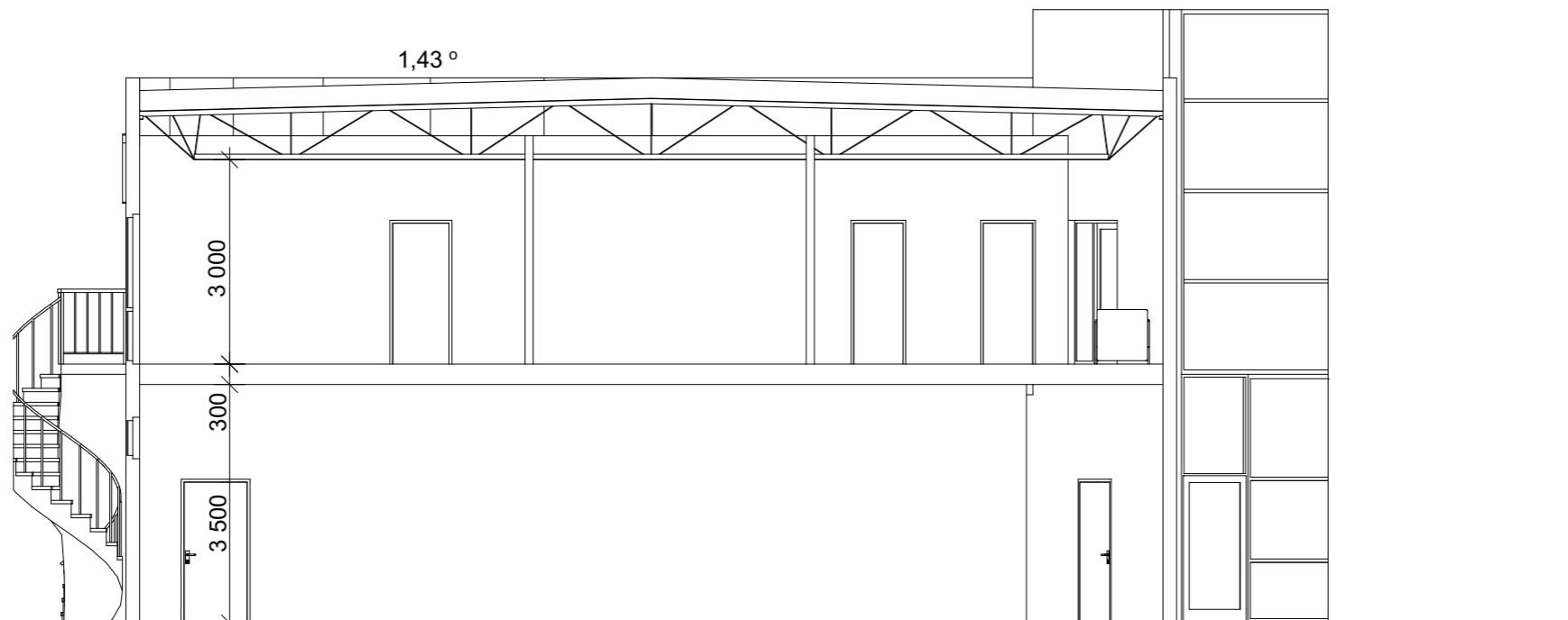
SEKTION A-A 1:100
