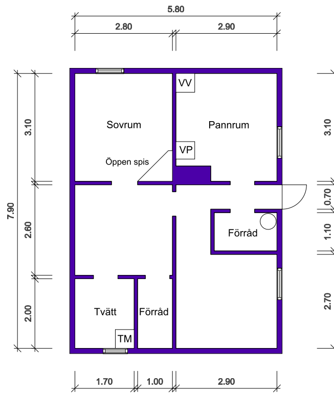
Källarplan
