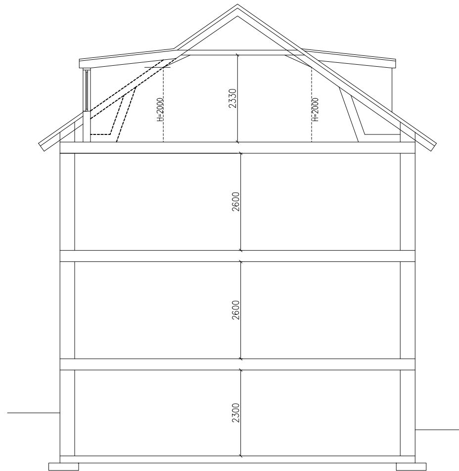
SEKTION A-A
