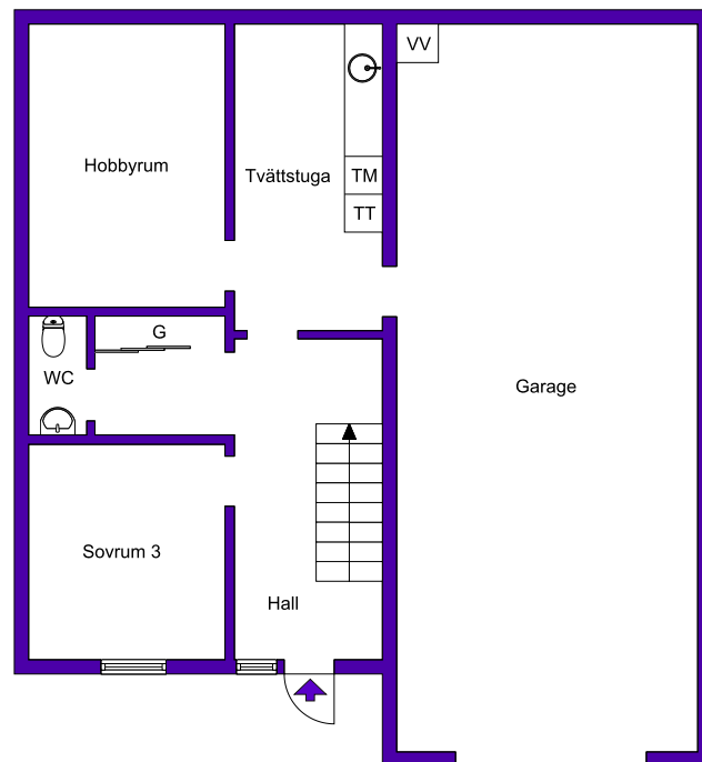
Souterrängplan
