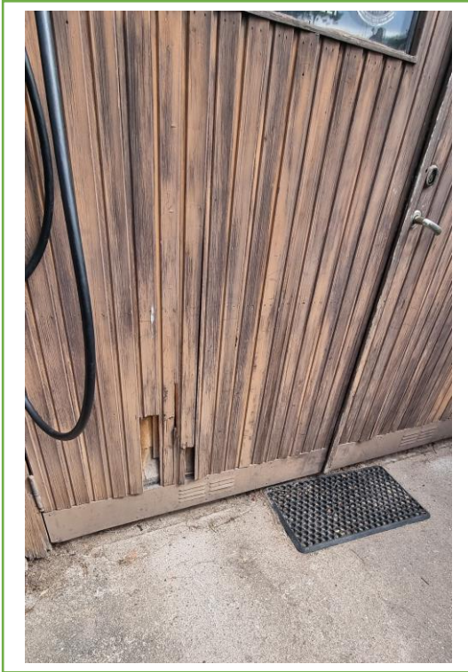
Bild 13: Rötskador på garagedörr.
