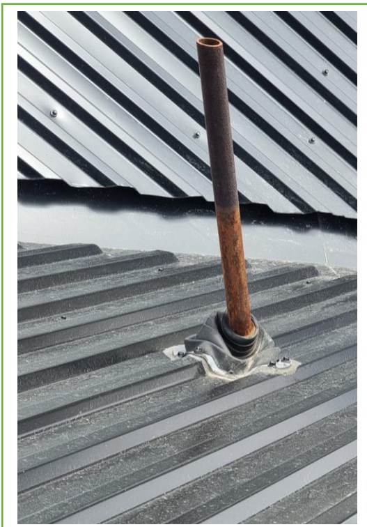
Bild 20: Otätt vid gummipackning till expansionskärl.
