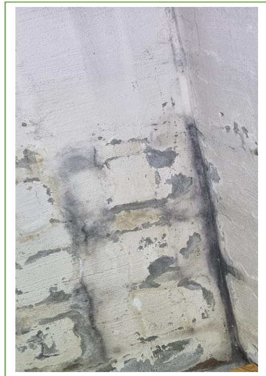
Bild 2: Fuktskador med påväxt i källare mot garageuppfart
