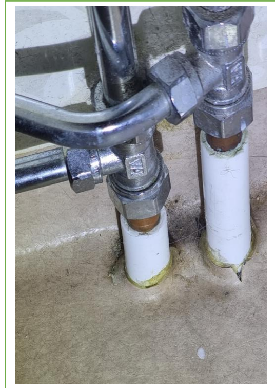
Bild 10: Otätt runt rörgenomföringar i golv (Badrum entréplan)
