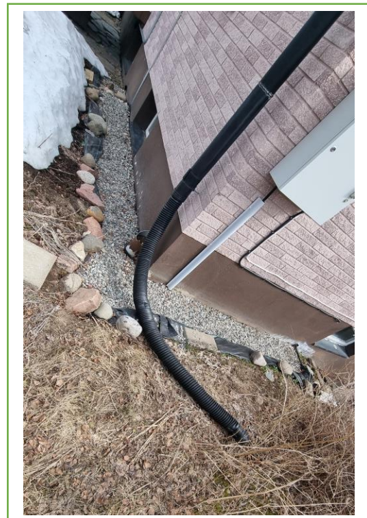
Bild 21: Dagvatten leds ej bort från grund.
