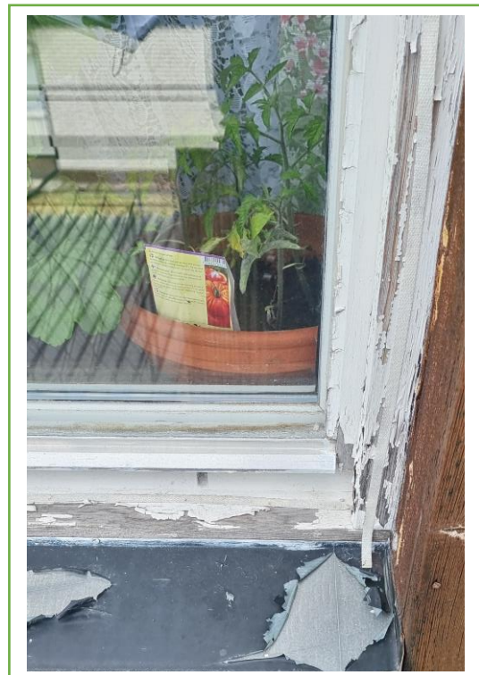
Bild 12: Kitt och färgsläpp på fönster.
